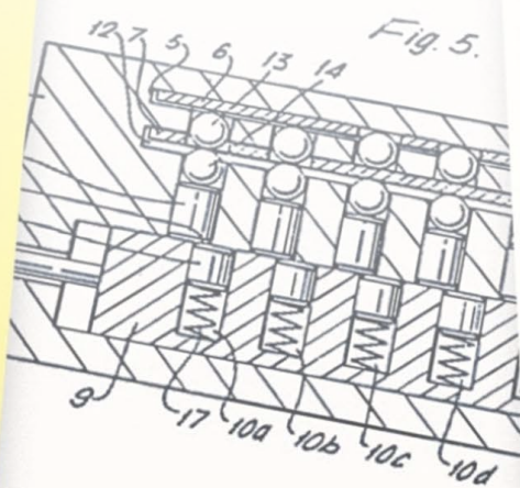
Den første prototypen på VingCard låsen.
